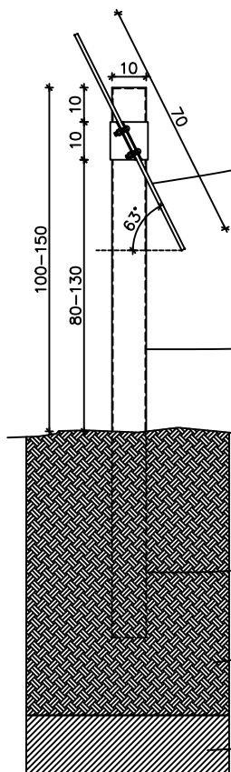
חתך א' כלא קנ"מ
