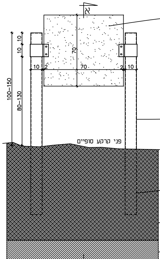
חזית כלא קנ"מ
