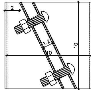
מחבר כלוח אלומיניום 10מ"מ
