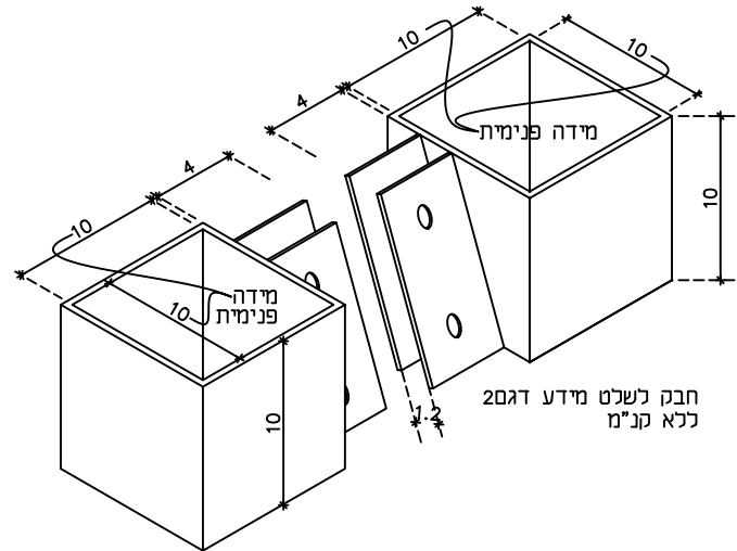
מחבר כלוח אלומיניום 10מ"מ
