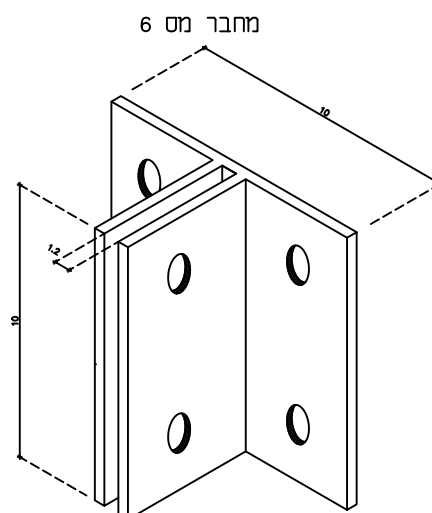
מחברים צמודי דופן
