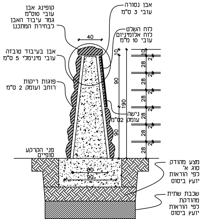
מסד עם חיפוי אבן חתך ב' ללא קנ"מ
